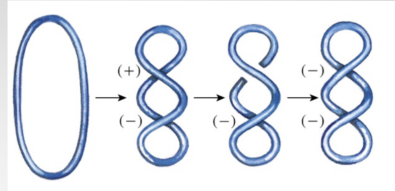
Mécanisme d'action de la gyrase sur un ADN circulaire
